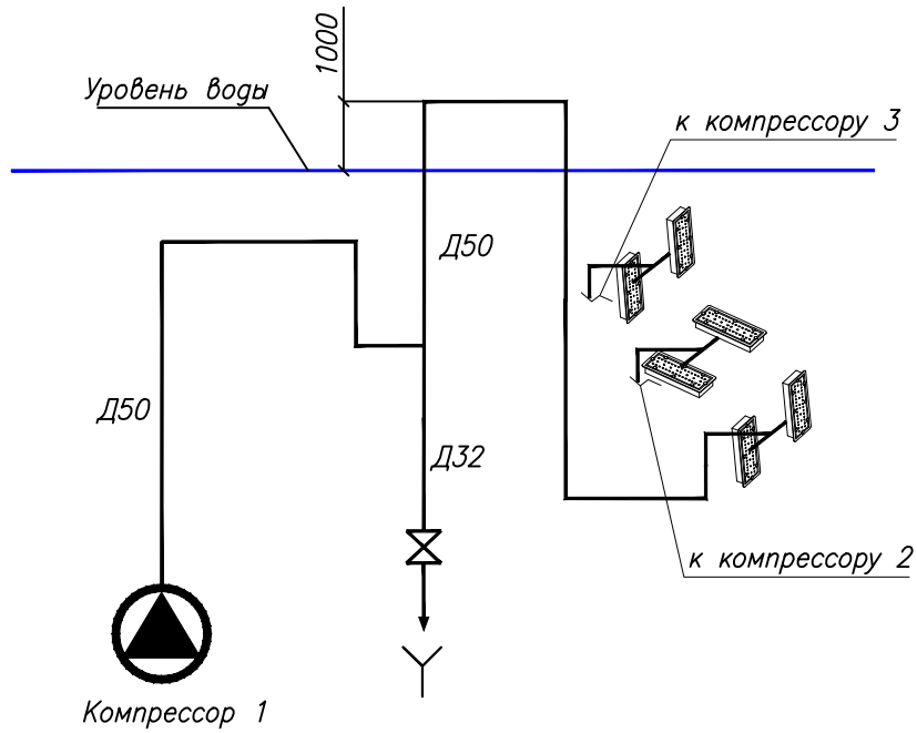
Водопад
