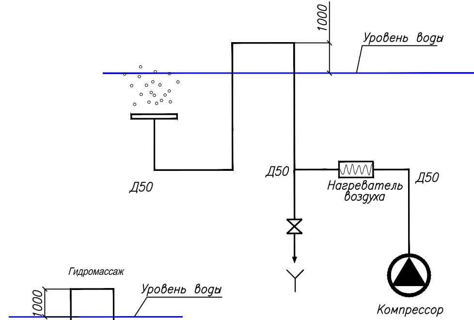
Гейзер
